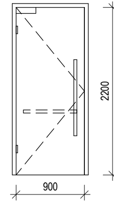
D06 Dveře jednokřídlé, otevírací, plné Dveře vedoucí do wc ZTP
