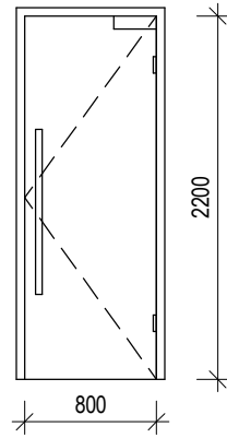
D04 Dveře jednokřídlé, otevírací, plné D05 Dveře vedoucí do wc předsíně
