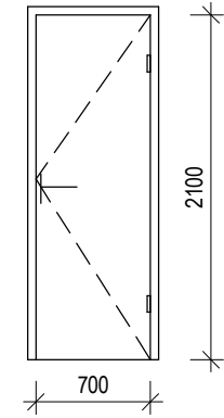
D08 Dveře jednokřídlé, otevírací, plné
