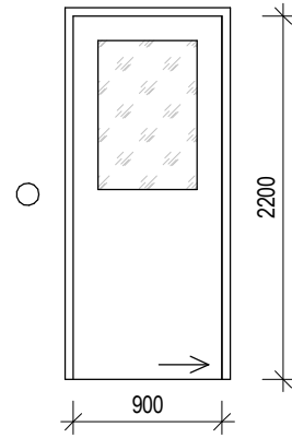
D02 Dveře jednokřídlé, posuvné, prosklené D03 Dveře vedoucí do kuchyně
