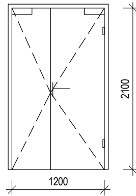
D22 Dveře jednokřídlé, otevírací, plné Dveře vedoucí do rozvodny ze vstupní haly.
