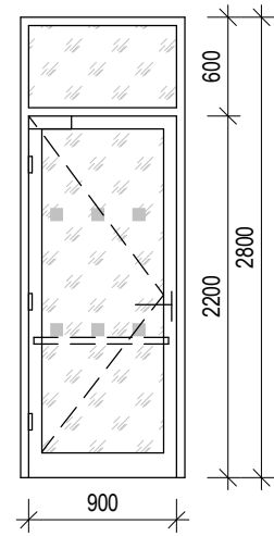
D01 Dveře jednokřídlé, otevírací, prosklené, s nadsvětlíkem Dveře vedoucí z restaurace do vstupní haly
