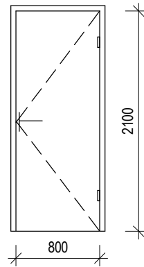
D18 Dveře jednokřídlé, otevírací, plné D20
