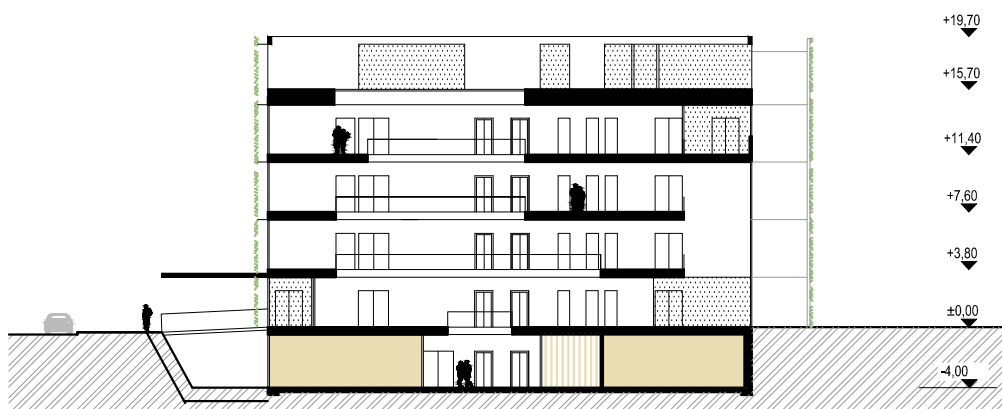
PŘÍČNÝ ŘEZ VSTUPNÍ DVORANOU
