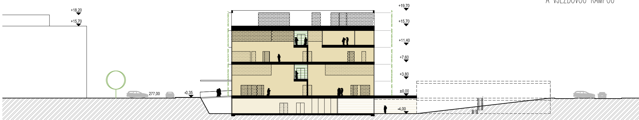
PŘÍČNÝ ŘEZ VÝROBOU A VJEZDOVOU RAMPOU
